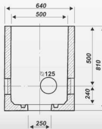
Przekrój poprzeczny
